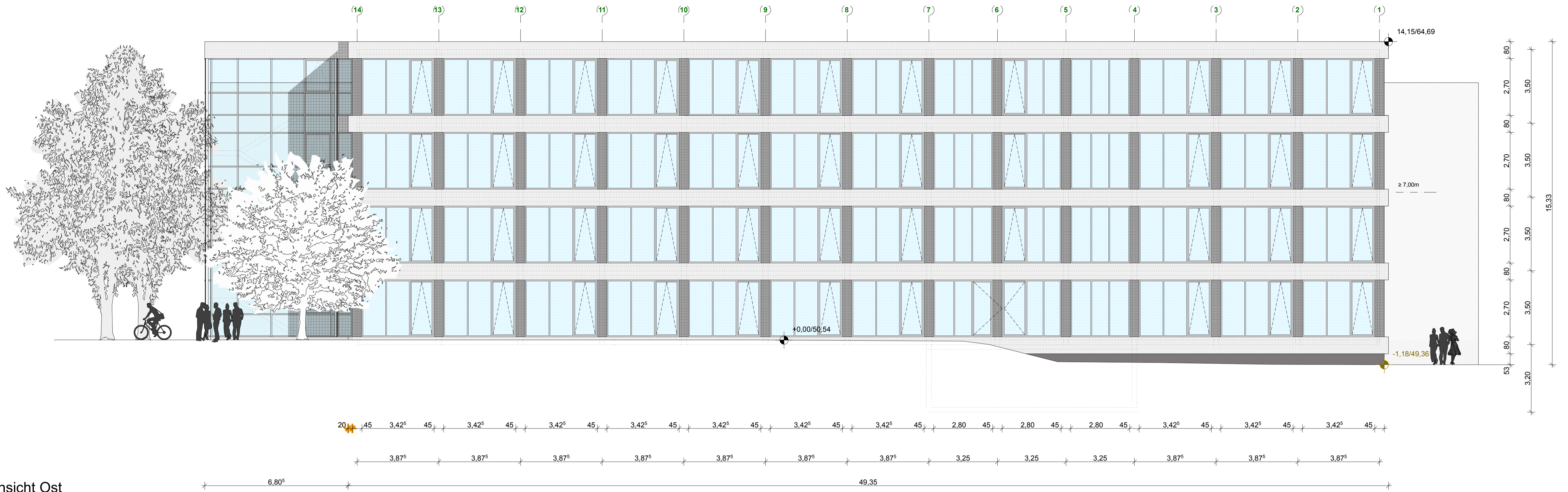
Ansicht Ost
